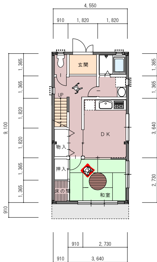
1 F 平面図
